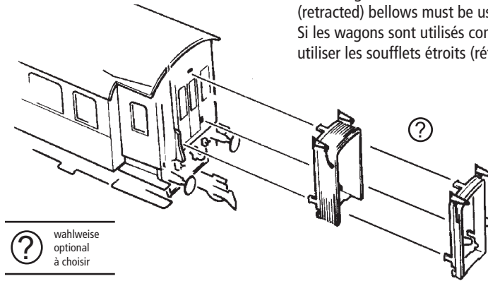
Dachabnahme / Steckteile Removal of roof / Extra parts Démontage du toit/ Pièces de finition
